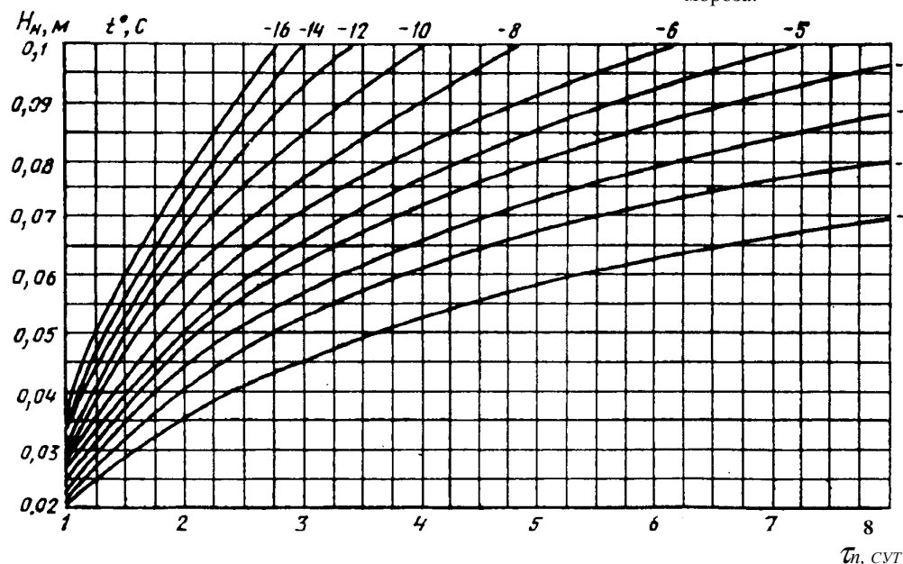
Рис. 7. Зависимость глубины промораживания слоя осадка от среднесуточной температуры воздуха и продолжительности промораживания
