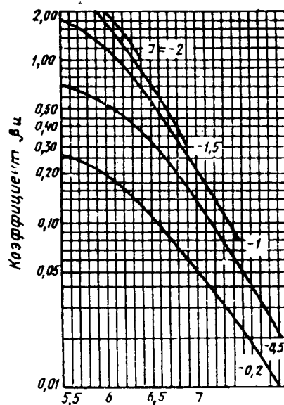
Рис. 4. Номограмма для определения коэффициента \beta_{\text{и}} при расчете дозы щелочи
