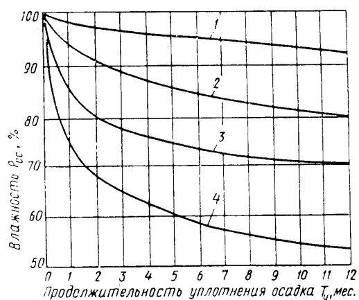
Рис. 4. Средние значения влажности осадка станций обезжелезивания и реагентного умягчения воды при уплотнении до одного года
